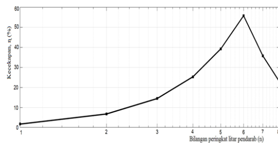
RAJAH 6. Kecekapan terhadap bilangan peringkat litar pendarab
