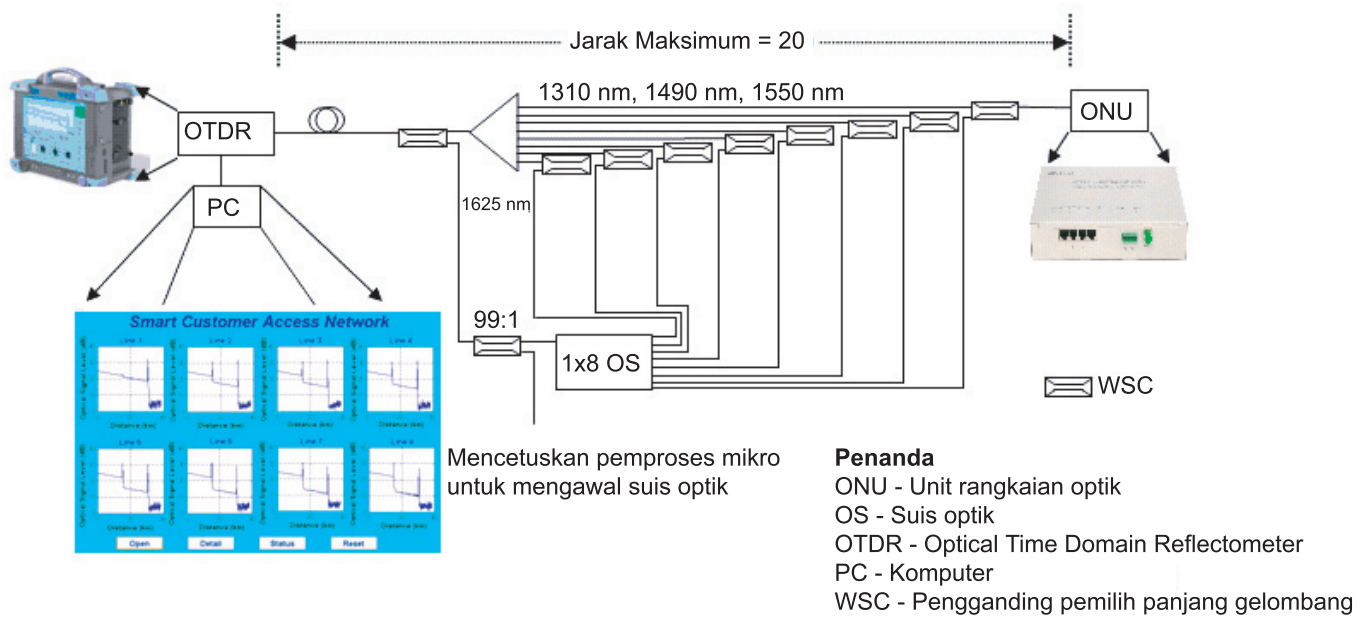
Rajah 2. Skema cadangan penyambungan suis optik kepada sistem pencerai dan pemproses mikro
